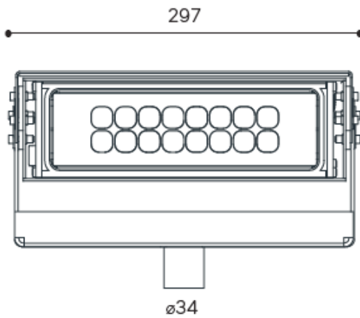
Frontansicht
