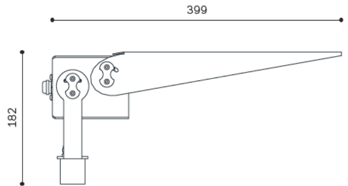
Seitenansicht
