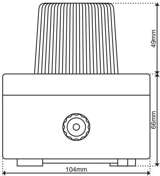
Seitenansicht
